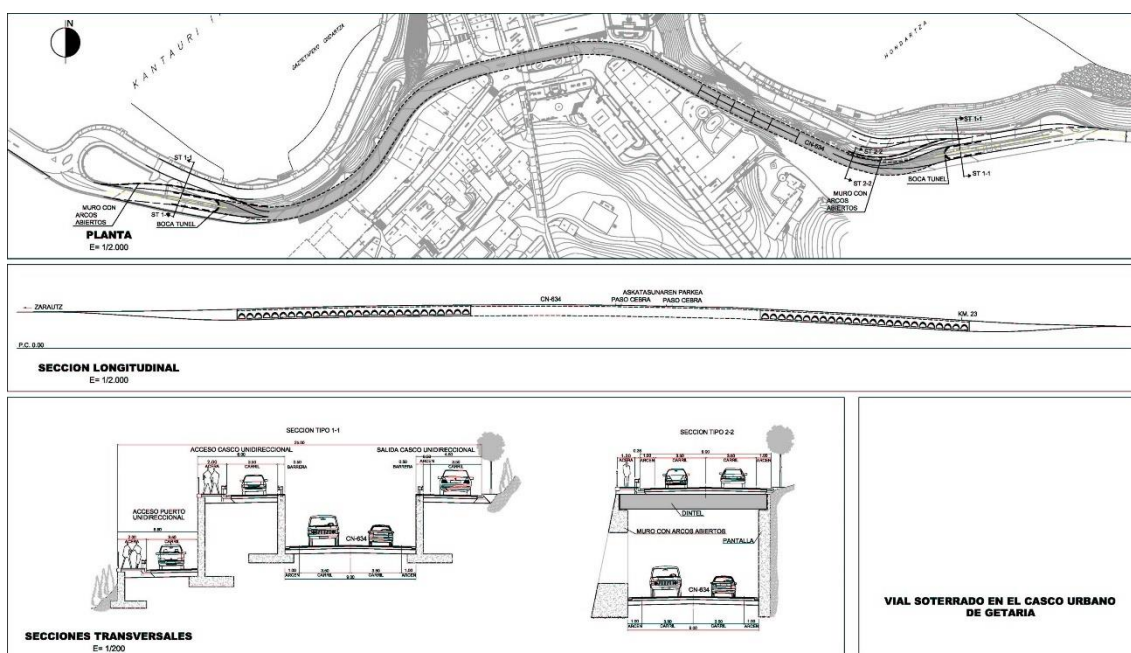
N-634 errepidearen trazadurari buruz udalerrian zehar indarrean dagoen Planaren proposamena.
